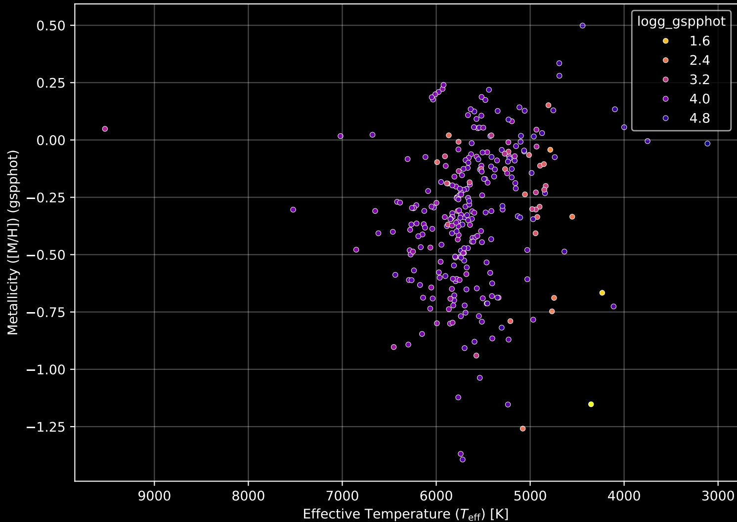
GALAH DR4 Field: [327] Stellar Population Parameters (n= 287)
